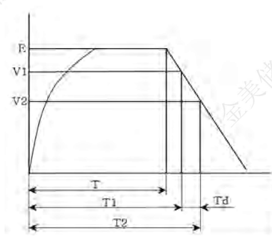
图2 样品的充放电曲线
